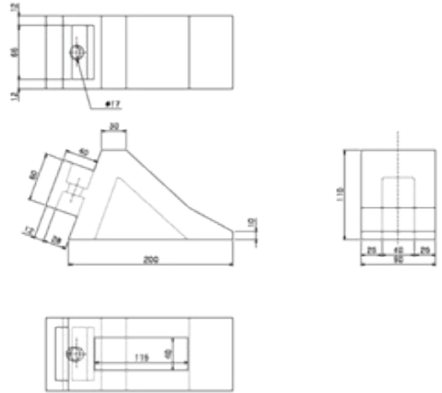
輪止め小
