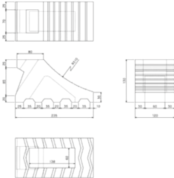
輪止め大
